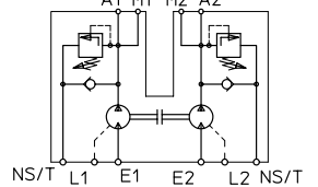
Circuit according DIN ISO 1219
